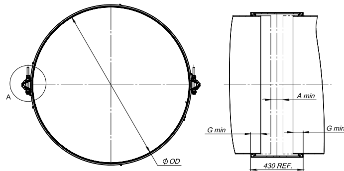
חבקים הידראוליים בקטרים נומינליים 700 מ"מ - 1,950 מ"מ, רוחב 430
