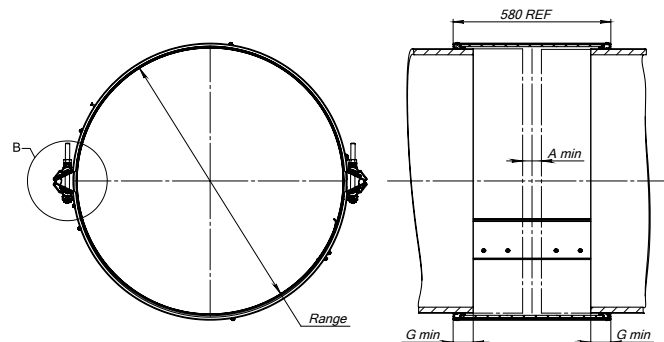
חבקים הידראוליים בקטרים נומינליים 700 מ"מ - 1,950 מ"מ, רוחב 580
